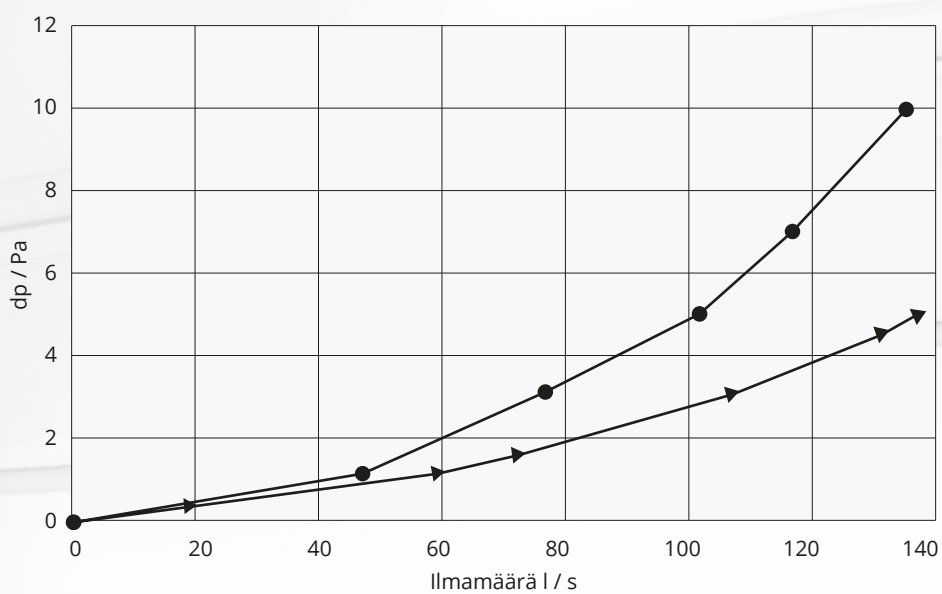
Painehäviö d160
